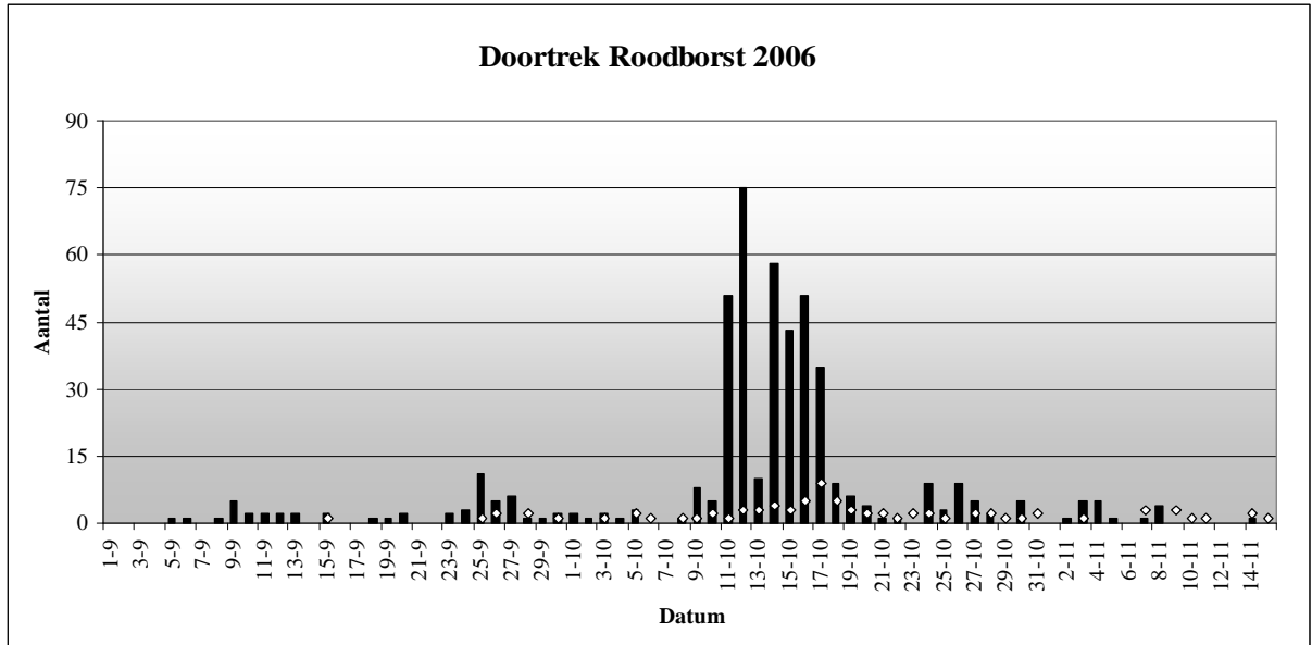
Figuur 6. Ring- en terugvangaantallen Roodborst 2006.
