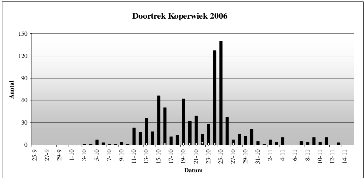
Figuur 7. Ring- en terugvangaantallen Koperwiek 2006.
