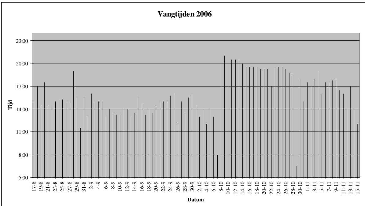
Figuur 2. Vangtijden "Ringgroep Derde KP Vlieland" 2006.
