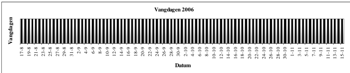
Figuur 1. Vangdagen "Ringgroep Derde KP Vlieland" 2006.
