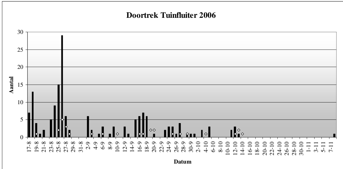
Figuur 5. Ring- en terugvangaantallen Tuinfluiter 2006.
