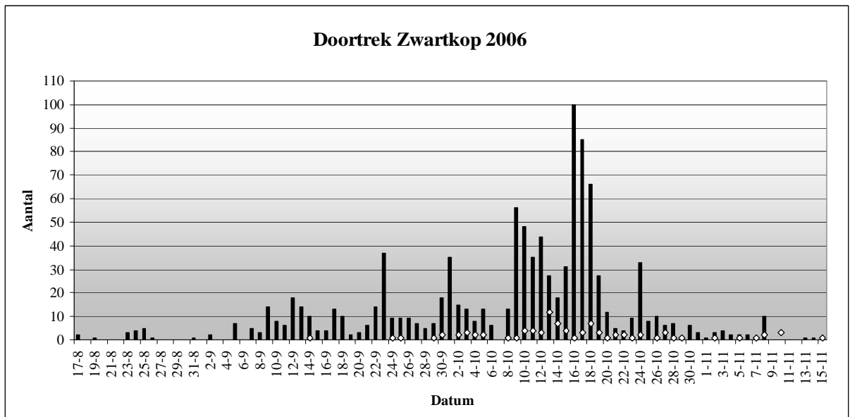
Figuur 4. Ring- en terugvangaantallen Zwartkop 2006.
