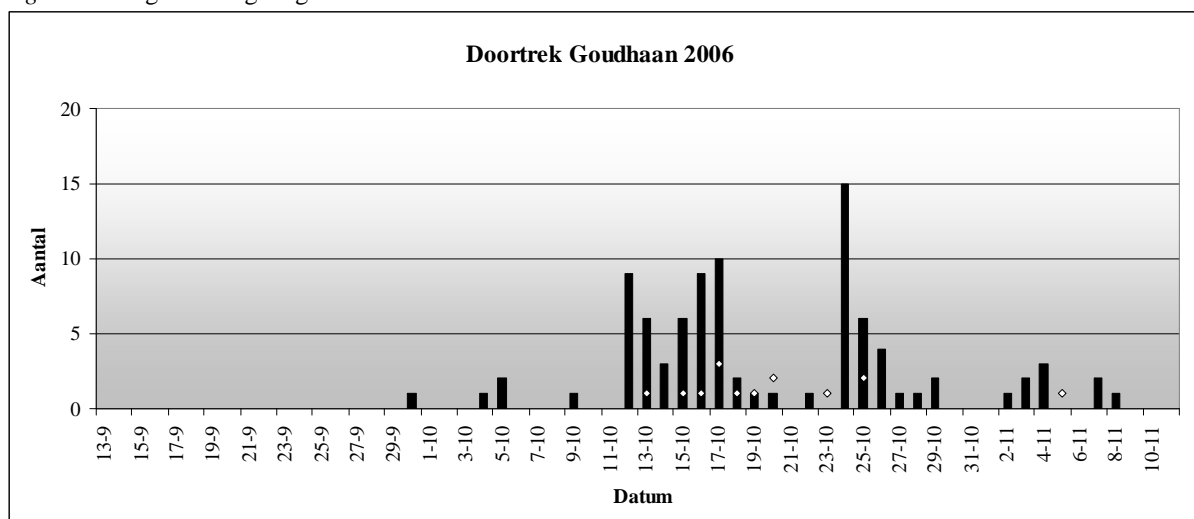
Figuur 3. Ring- en terugvangaantallen Goudhaan 2006.
