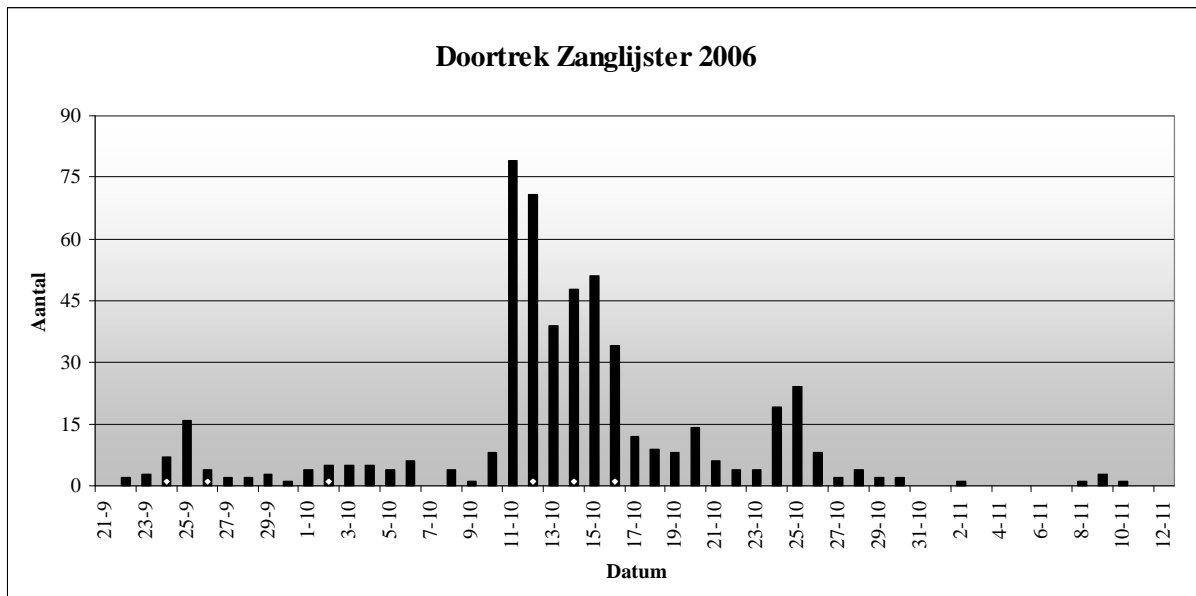
Figuur 8. Ring- en terugvangaantallen Zanglijster 2006.
